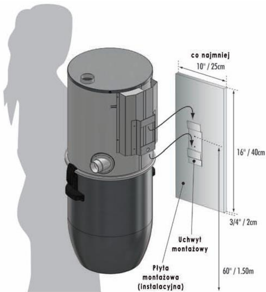
Rys. 1. Uchwyt montażowy
