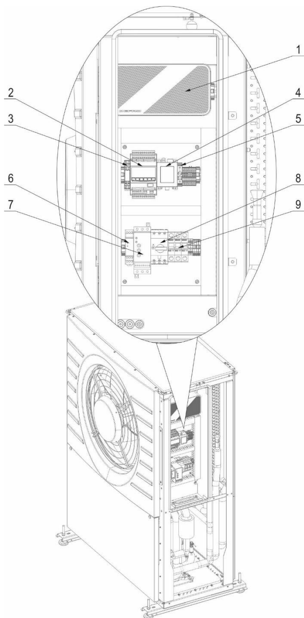
Rysunek 3. Sterownik obiegu chłodniczego w jednostce zewnętrznej. 1-sterownik obiegu chłodniczego; 2-przełącznik; 3-sterownik zaworu rozprężnego; 4-transformator napięcia; 5-bezpiecznik STB; 6-czujnik kontroli i zaniku fazy; 7-soft-start; 8-wyłącznik silnikowy sprężarki; 9-wyłącznik nadprądowy.
