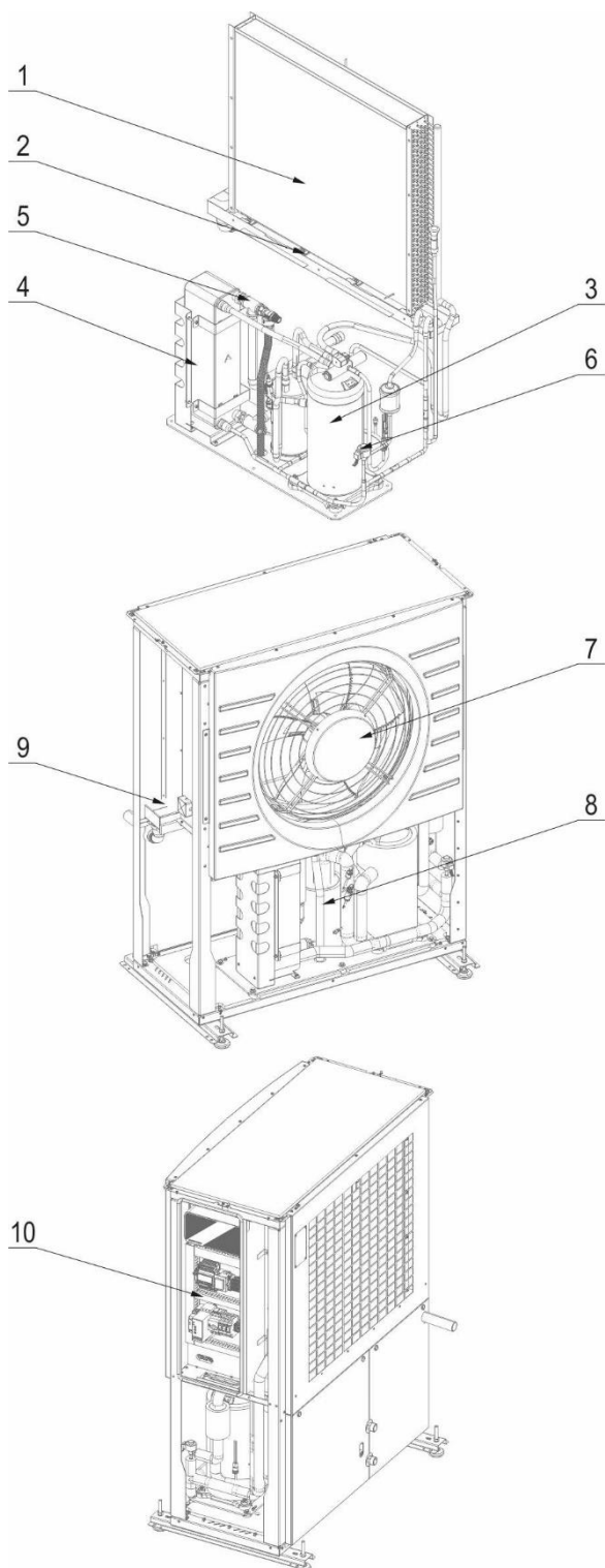
Rysunek 1. Jednostka zewnętrzna.
