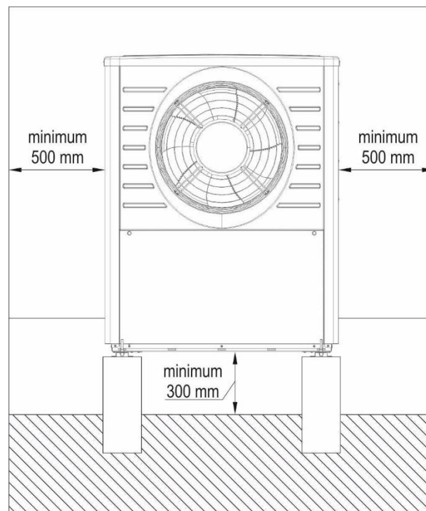
Rysunek 7. Miejsce montażu pompy ciepła rzut przodu.
