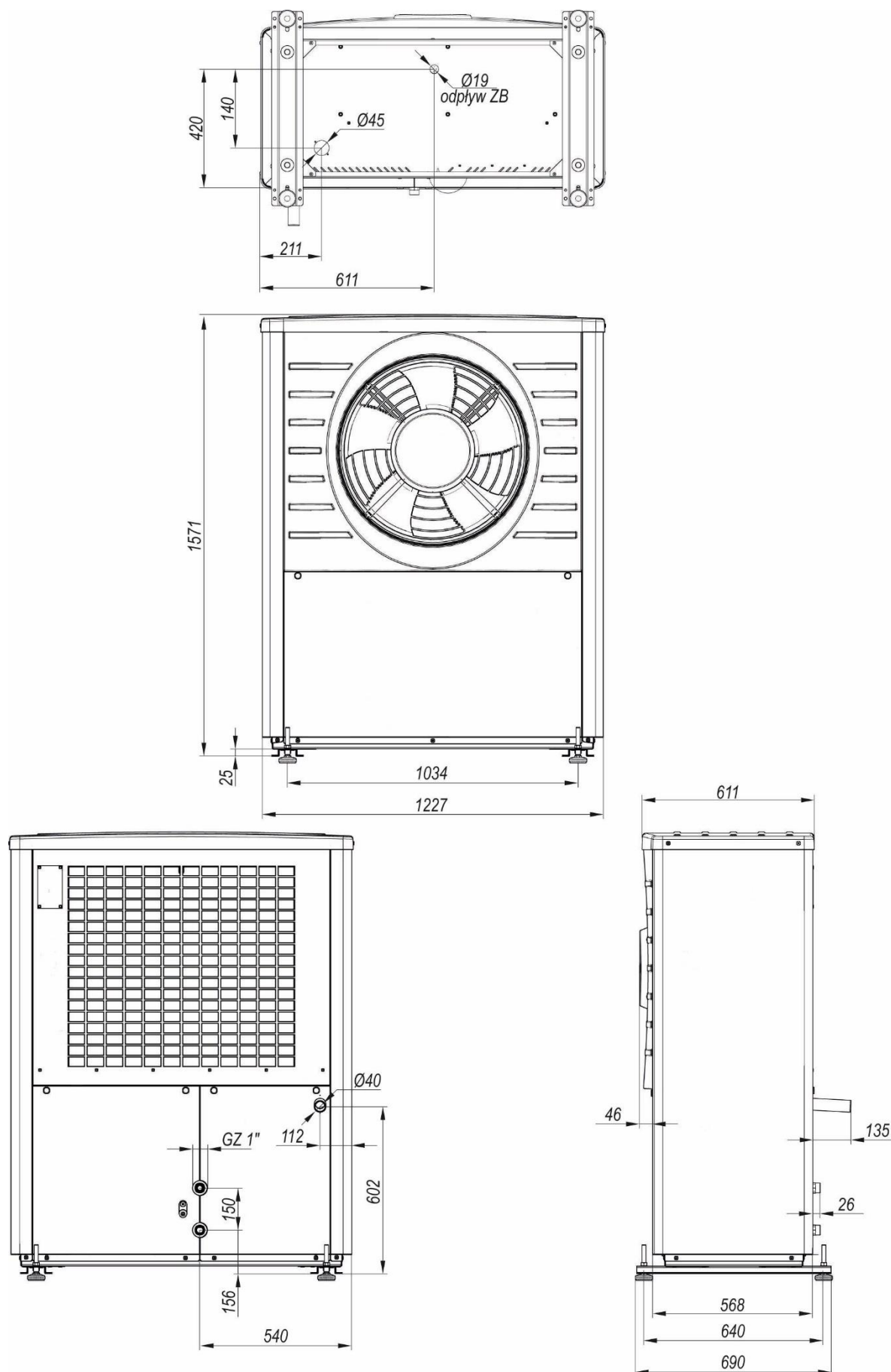
Rysunek 10. Wymiary jednostki zewnętrznej – TOP VAC R290V VERTICAL 8 i TOP VAC R290V VERTICAL 12
