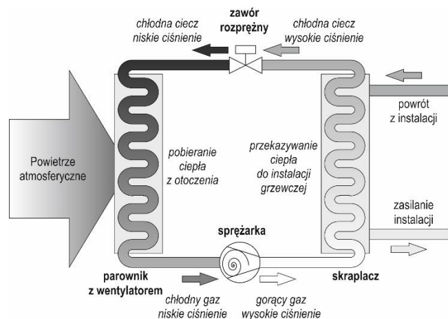
Rysunek 2. Zasada działania pompy ciepła TOP VAC R290V VERTICAL.
