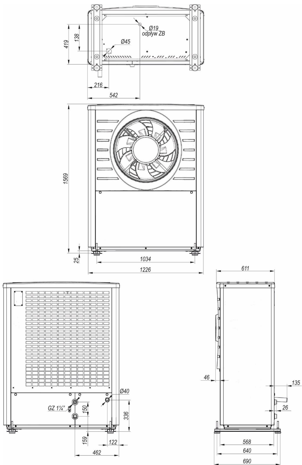
Rysunek 11. Wymiary jednostki zewnętrznej – TOP VAC R290V VERTICAL 16
